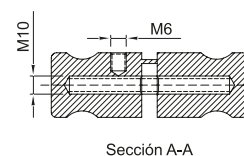
Sección A-A
