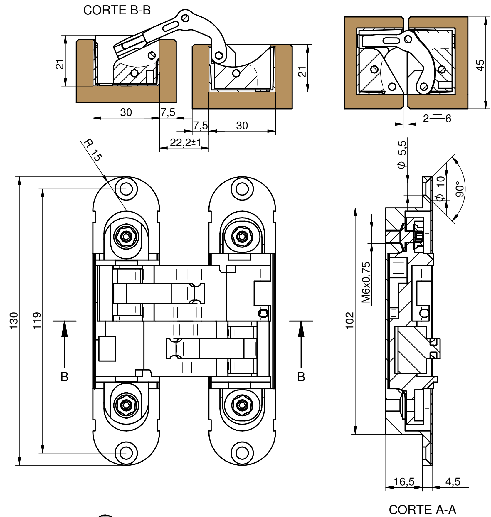
DETALLES TÉCNICOS DE BISAGRA
