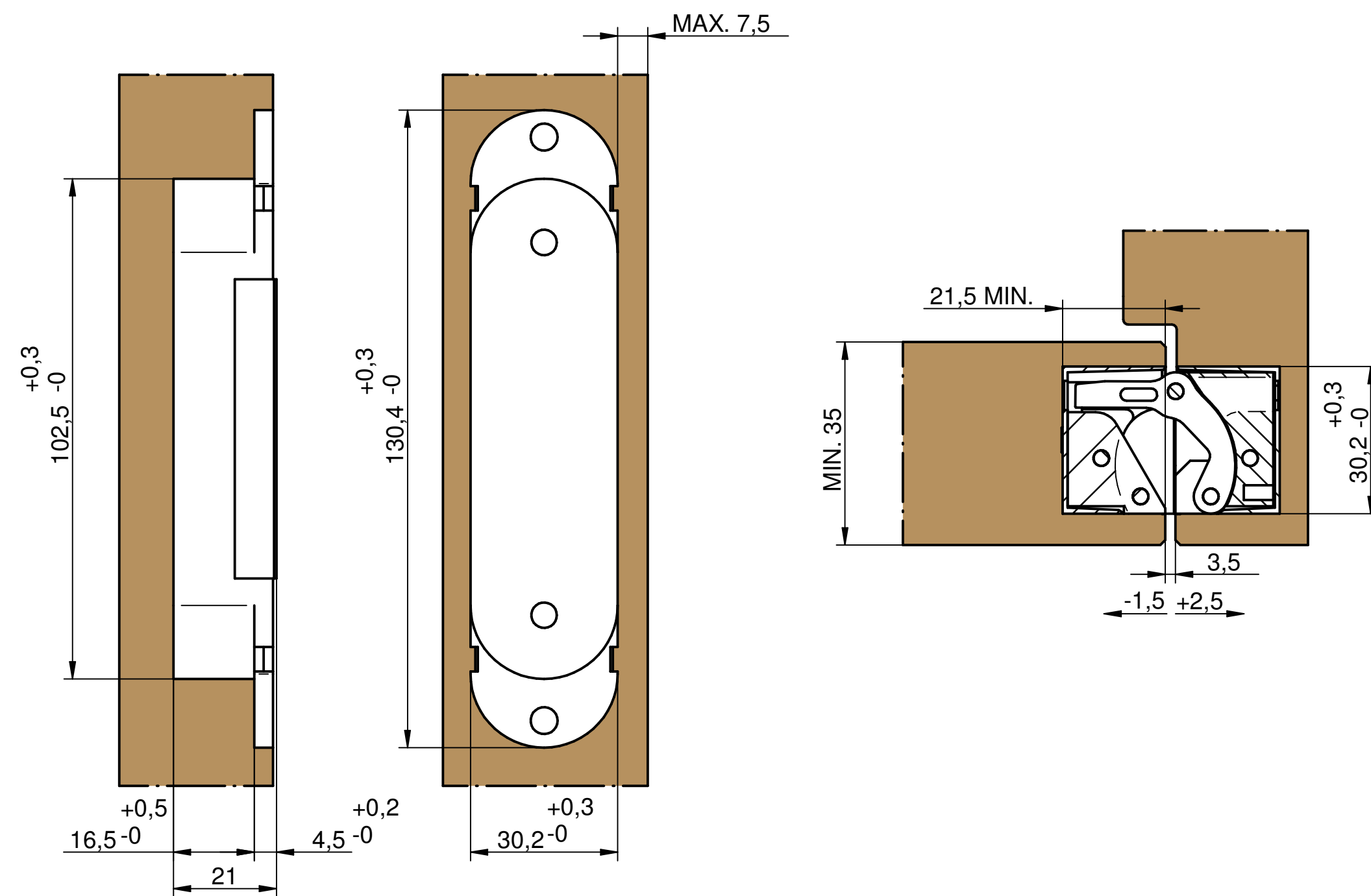
DETALLES TÉCNICOS MECANIZACIÓN DE PUERTA
