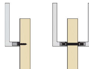
DETALLE FIJACIONES MADERA
