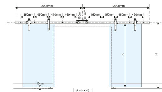
Montaje 2 Hojas
