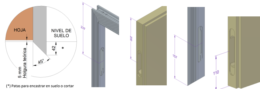
MARCO STANDARD CORTE INFERIOR 80 MM
