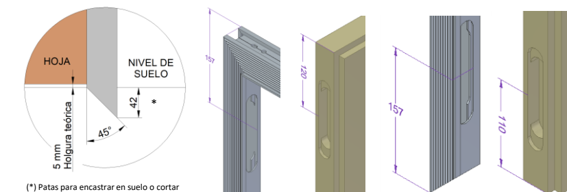
MARCO STANDARD CORTE INFERIOR 80 MM + CORTE SUPERIOR 80 MM
