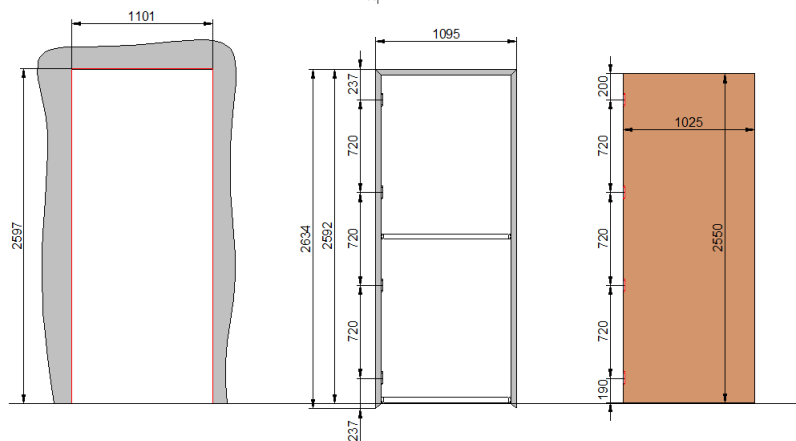
MARCO STANDARD CORTE INFERIOR 80 MM + CORTE SUPERIOR 80 MM
