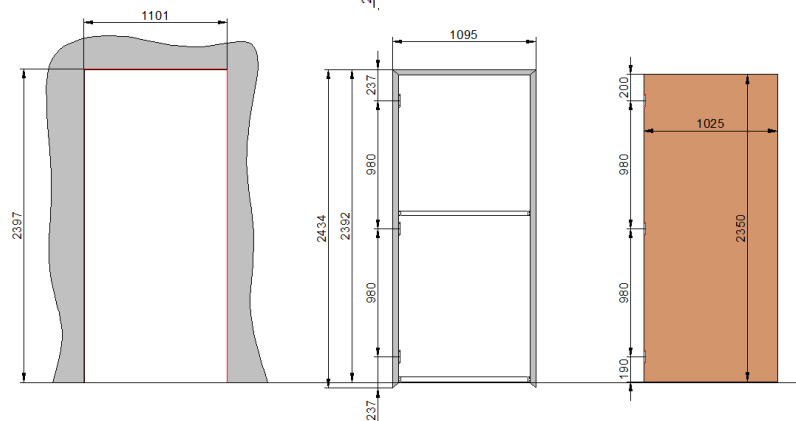
MARCO STANDARD CORTE INFERIOR 80 MM
