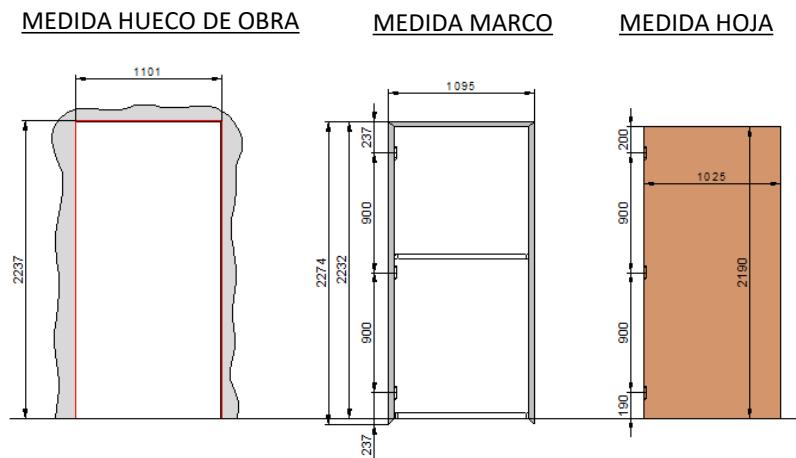
MARCO STANDARD SIN CORTAR
