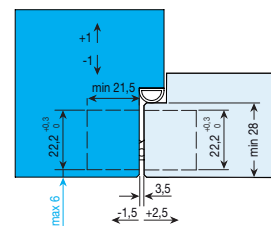
Sección puerta enrasada y solapada
