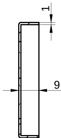
CORTE D-D
