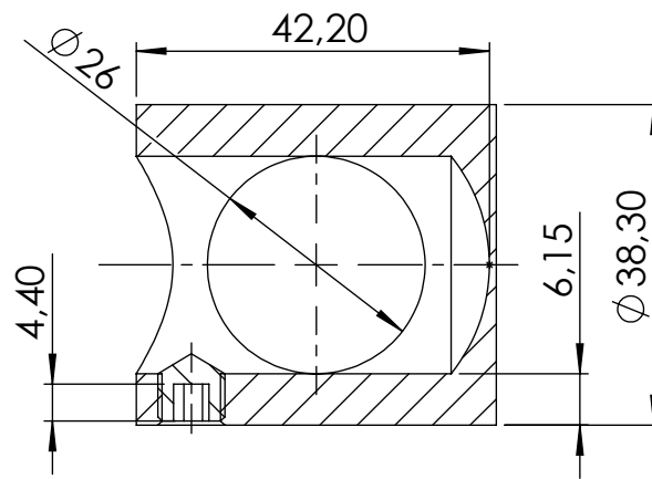
SECCIÓN A-A
