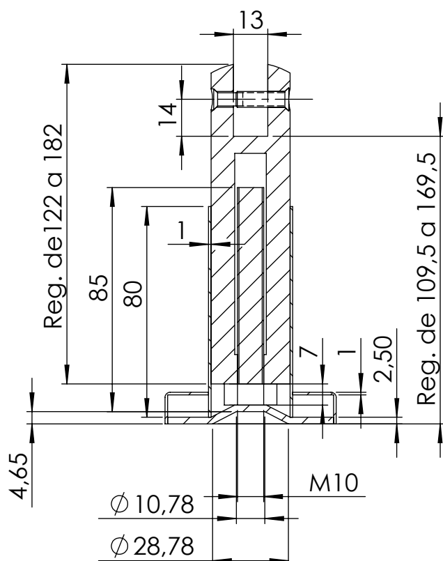
SECCIÓN A-A
