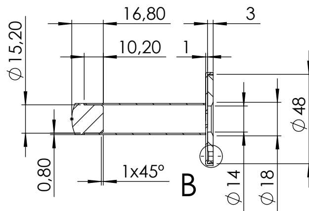
SECCIÓN A-A
