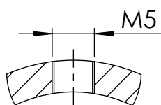
DETALLE A ESCALA 2 : 1
