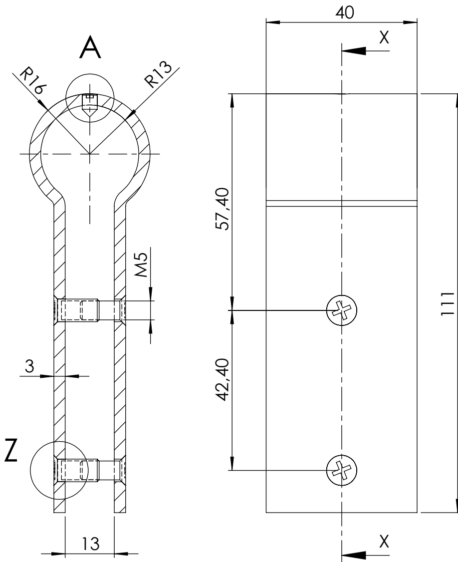
SECCIÓN X-X
